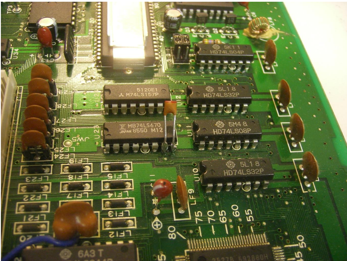
Condensator van 1nF tussen pin 7 en 8 van de 74LS670.
